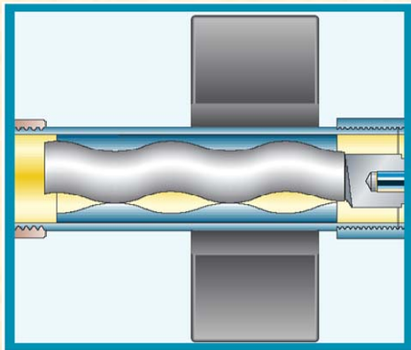
Rotore / Statore
